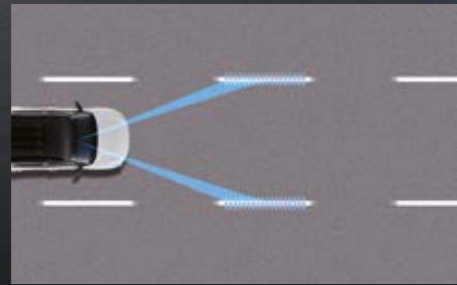
Sistema de permanencia en carril (LKAS) El LKAS puede detectar un cambio de carril inseguro (sin señalización previa) y corregir automáticamente la dirección para mantener el vehículo centrado en el carril correcto.
